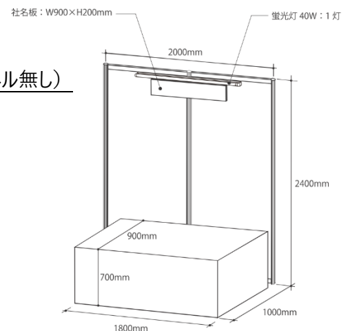
【基礎小間】
